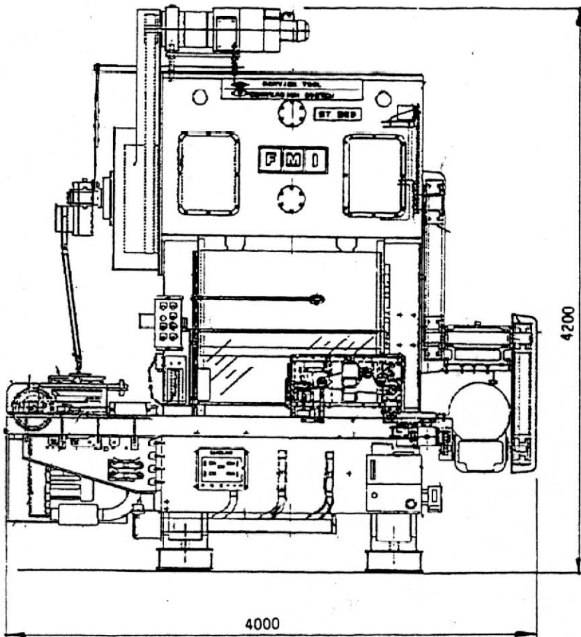
PRESSA mod. A790
